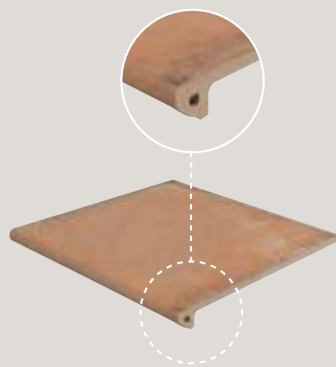
Peldaño Fiorentino 33 x 33 x 3 cm - 9.6" x 13.2" x 1.2"
